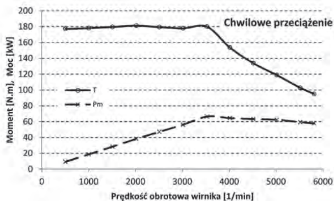
Rys. 4. Charakterystyki elektromechaniczne momentu T = f(n) i mocy na wale P_m = f(n) zmierzone w trakcie badań laboratoryjnych napędu E-Kit dla miejskiego samochodu osobowego
